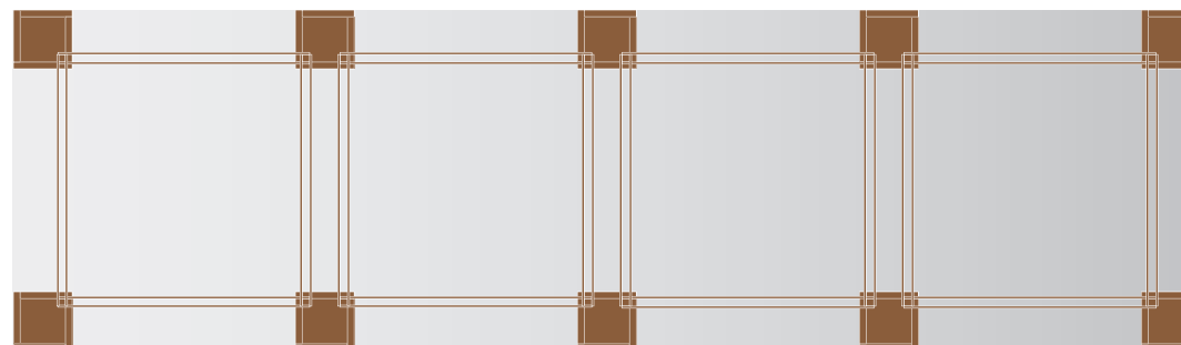
Variante XXL Durch die Außenpositionierung der Pflanzgefäße erhöht sich die Durchgangsbreite von 150 cm auf 265 cm. Ideal für Bänke und Tische, Liegen und vielem anderen. LxBxH in cm: 405/variabel x 405/variabel x 310
